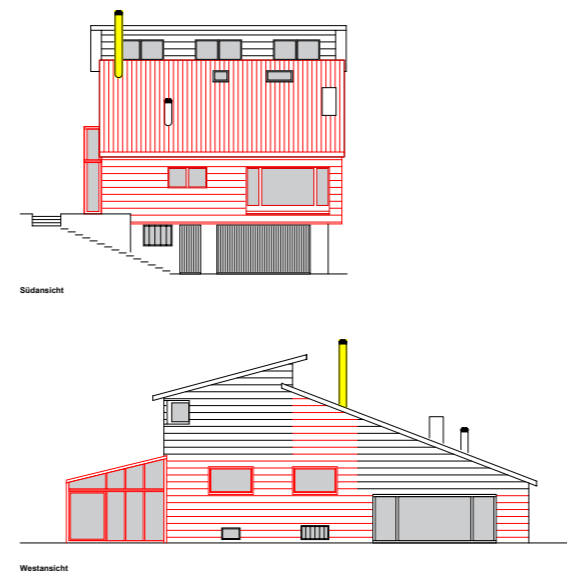
Umbau in zwei Etappen 2001/2008
