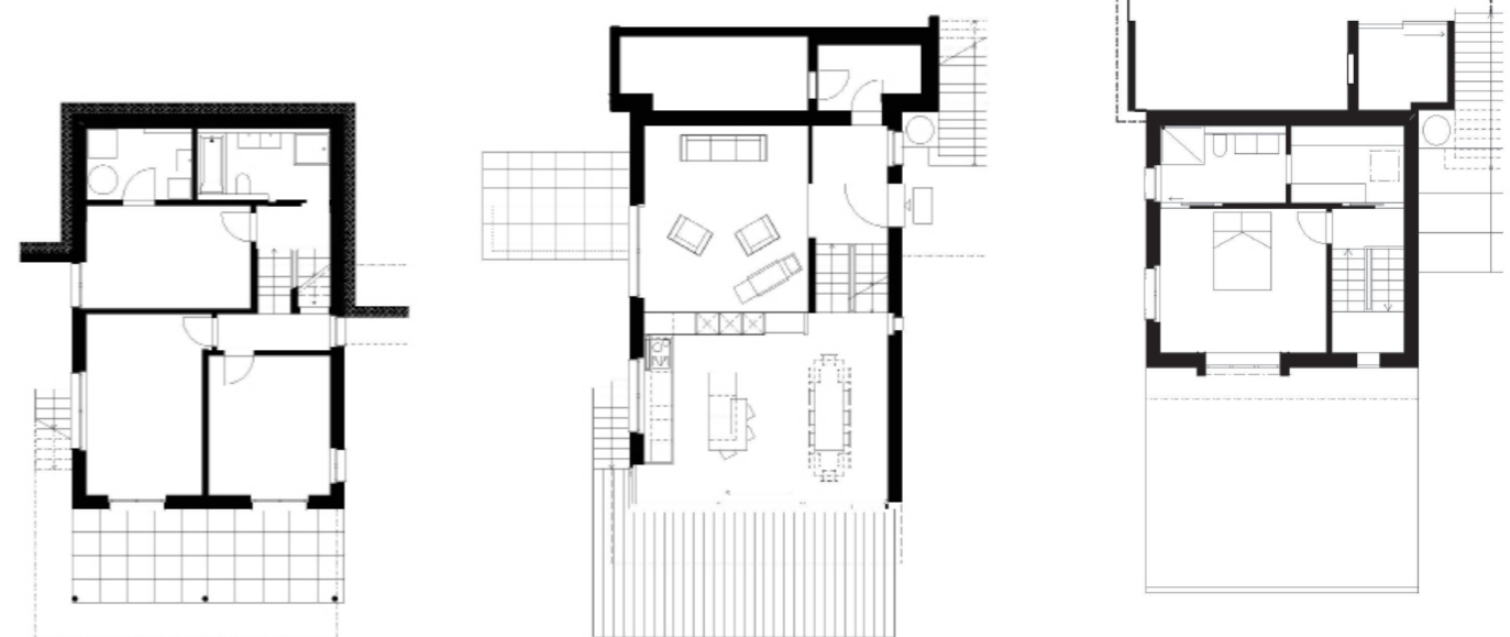
Untergeschoss
